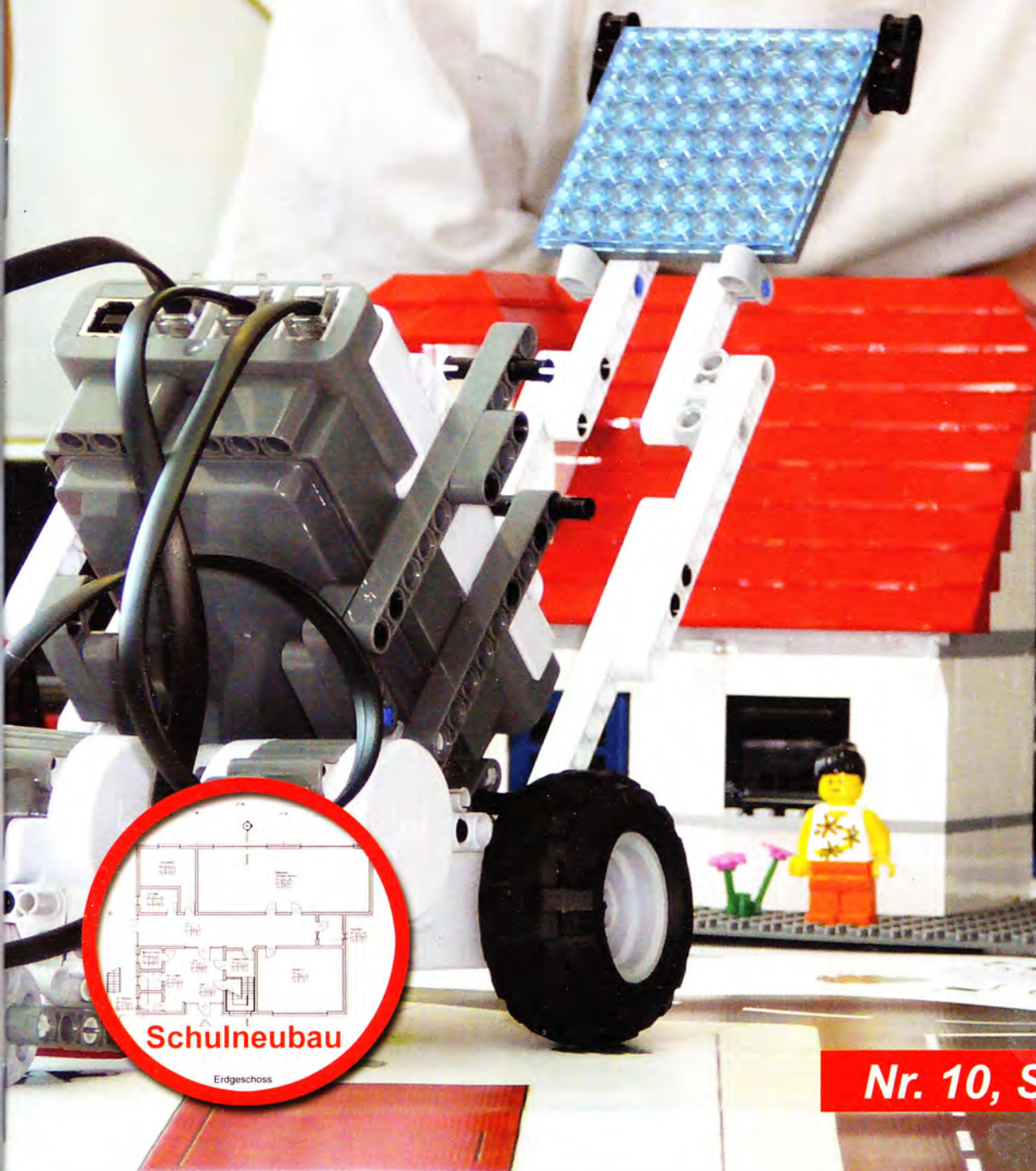
Roboter
